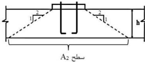
(ب) کفستون‌هایی که لبه‌های آن از لبه شالوده فاصله دارد
