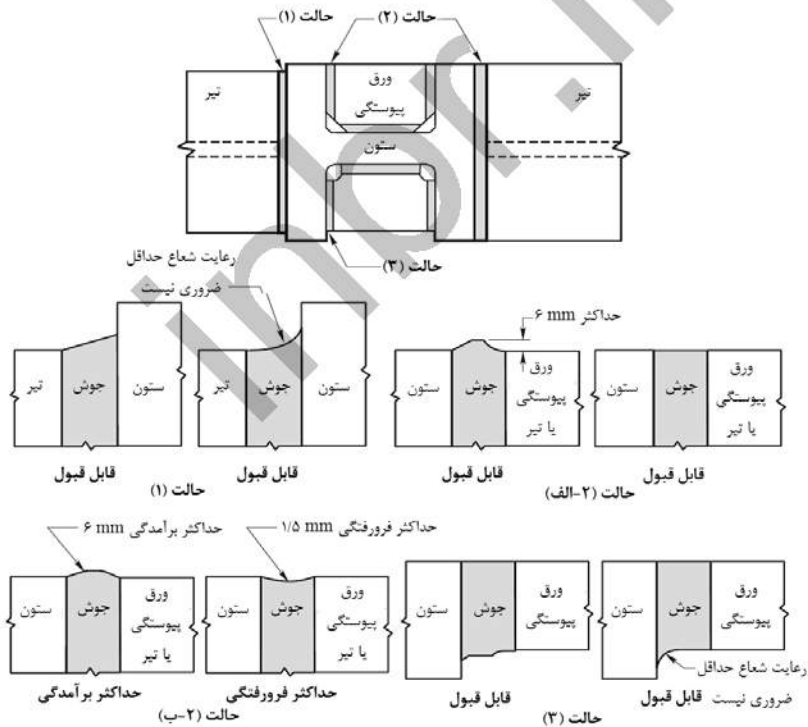
شکل ۴-۱۰-۴-۲۴: وضعیت‌های قابل قبول برداشتن ورق گوشواره‌ای (ناودان انتهایی جوش)
