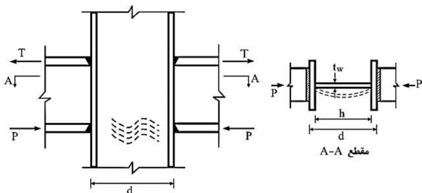
شکل ۱۰-۲-۹: کمانش فشاری جان در مقابل یک جفت نیروی متمرکز فشاری
