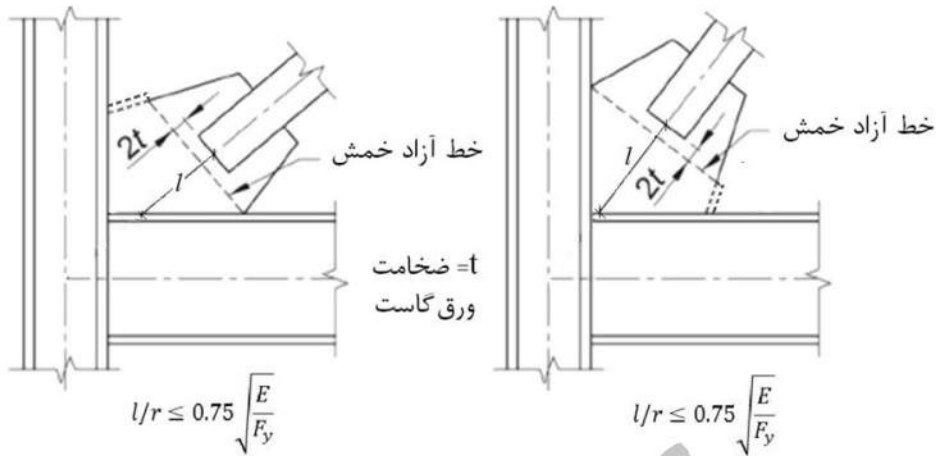
شکل ۳-۲-۴-۳-۱۰: سازگاری ورق اتصال (ورق گاست) با کمانش خارج از صفحه عضو مهاربندی
