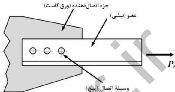
شکل ۱۰-۲-۱-۹: نام‌گذاری قسمت‌های مختلف یک اتصال
