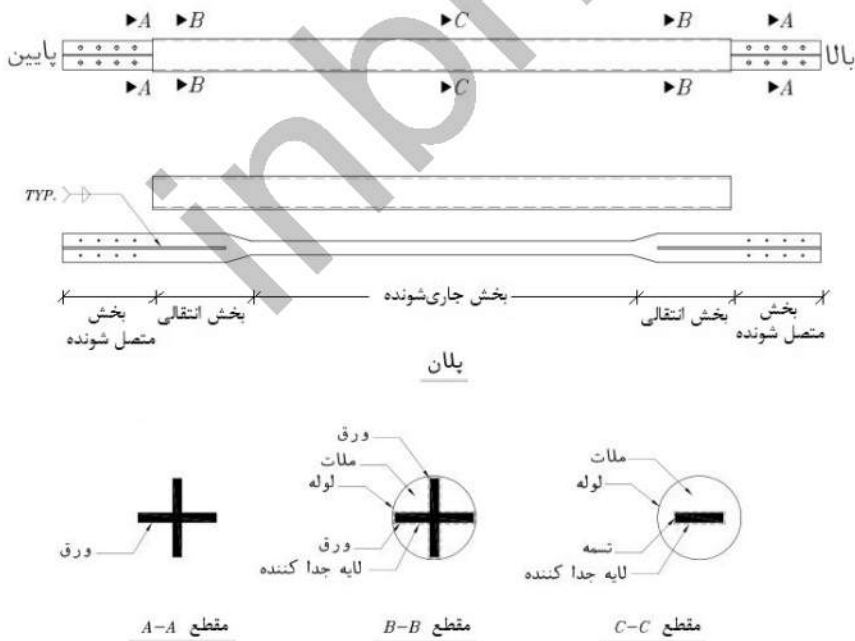
شکل ۳-۱۰-۴-۴-۳-۱۰: نمونه‌ای از اجزای یک مهاربند کمانش تاب
